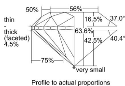
Profile to actual proportions
