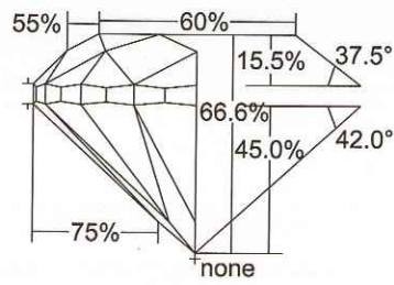
Profile to actual proportions
