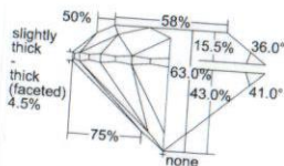
Profile to actual proportions
