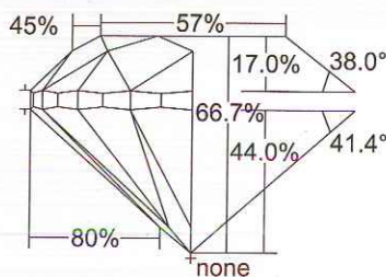
Profile to actual proportions
